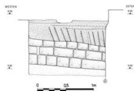
Abb. 297 F/I-1/19-Grab 1, Innenansicht der Nordwand
