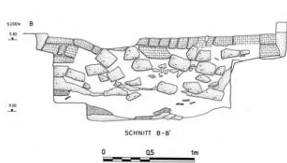
Abb. 294 F/I-1/19-Grab 1, Schnitt B-B'
