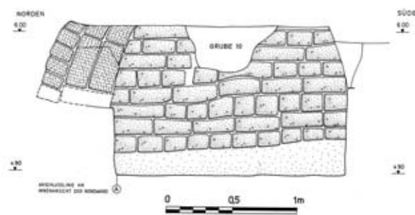
Abb. 296 F/I-1/19-Grab 1, Innenansicht der Grabeingangswand und Schnitt durch Gewölbe
