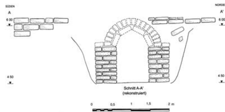
Abb. 288 F/I-1/19-Grab 6, Schnitt A-A'
