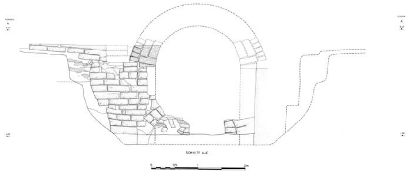
Abb. 293 F/I-1/19-Grab 1, Schnitt A-A'
